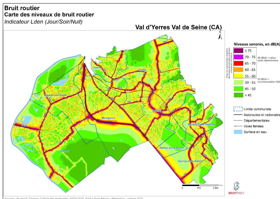
Figure 15a : Carte de type A – Bruit routier - Indicateur Lden
