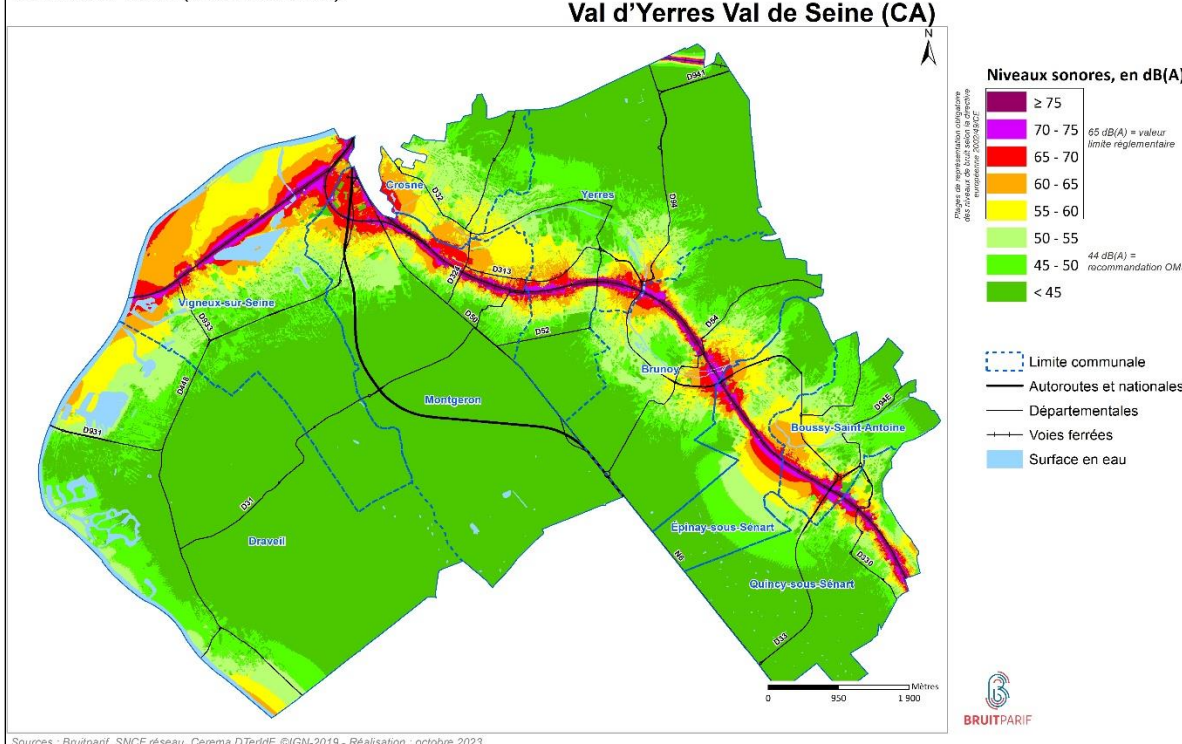
Figure 16a : Carte de type A – Bruit ferré - Indicateur Lden
