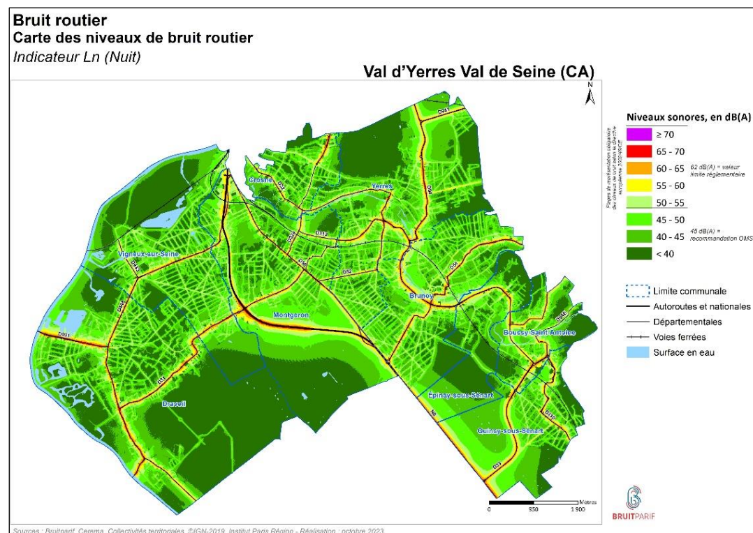
Figure 15b : Carte de type A – Bruit routier - Indicateur Ln
