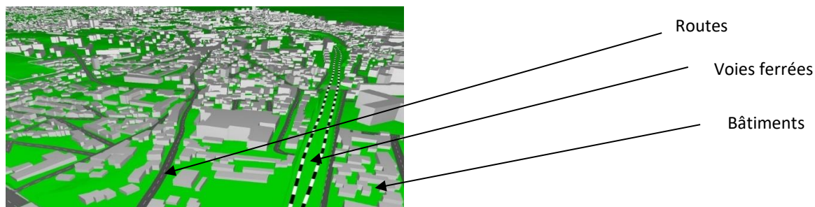
Figure 12 : Représentation 3D du modèle de calcul acoustique
