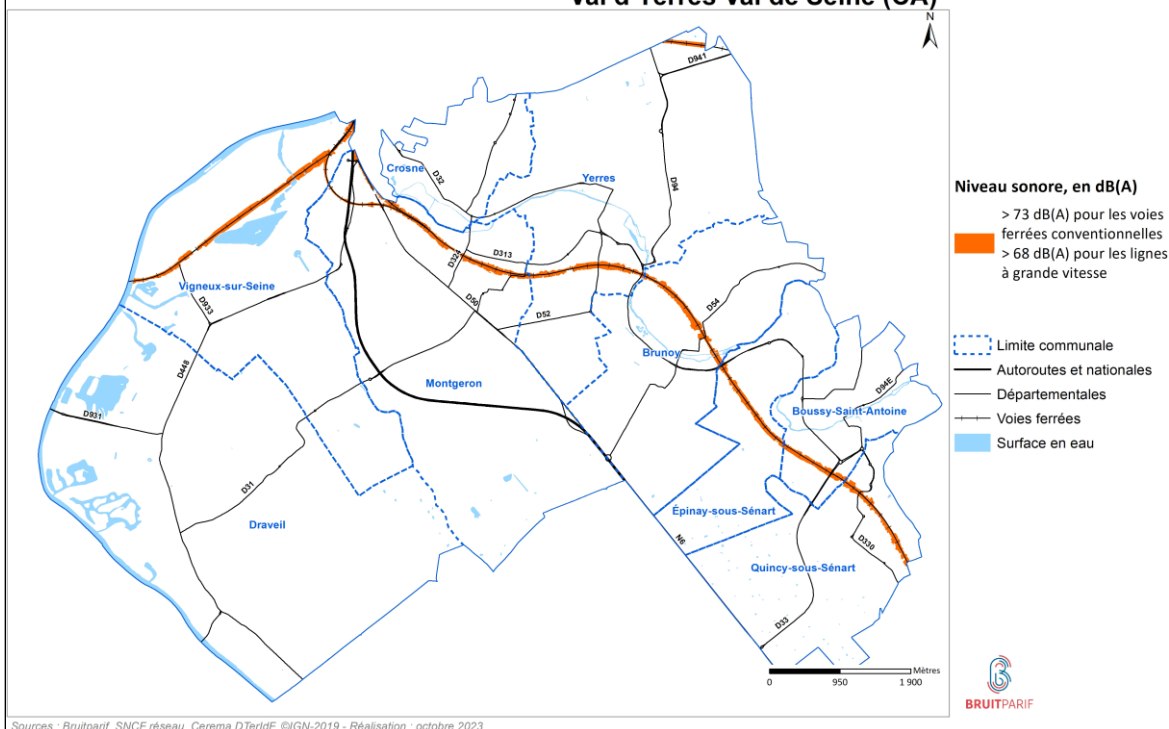
Figure 16c : Carte de type C – Bruit ferré - Indicateur L_{den}
