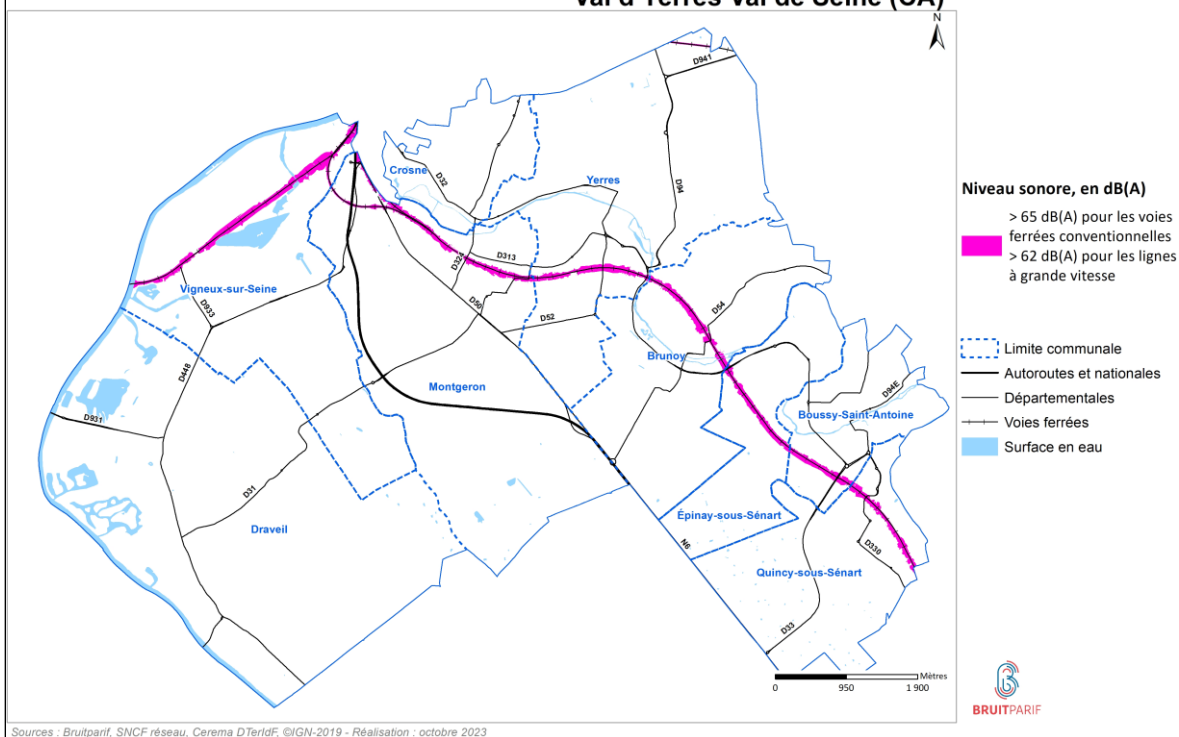
Figure 16d : Carte de type C – Bruit ferré - Indicateur L_n
