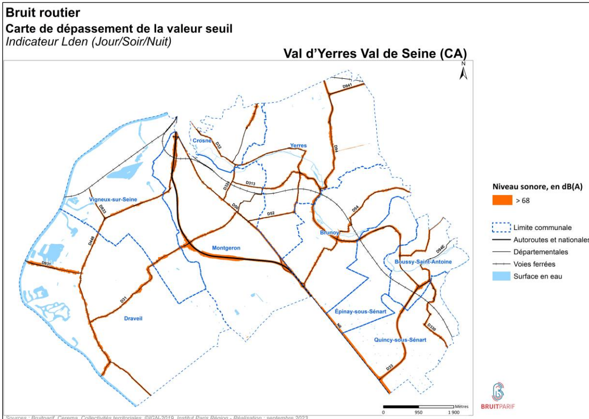
Figure 15c : Carte de type C – Bruit routier - Indicateur Lden
