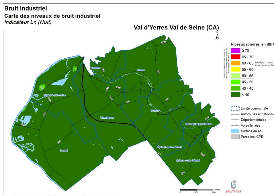
Figure 18b : Carte de type A – Bruit industriel - Indicateur Ln
