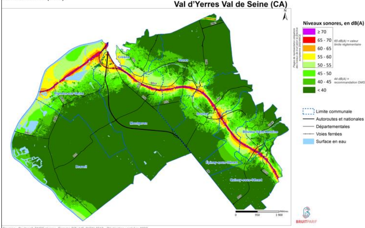
Figure 16b : Carte de type A – Bruit ferré - Indicateur Ln
